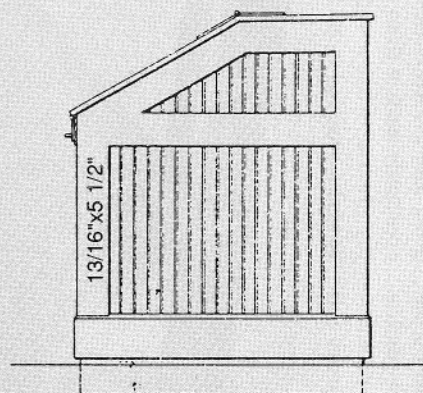
End Elevation
